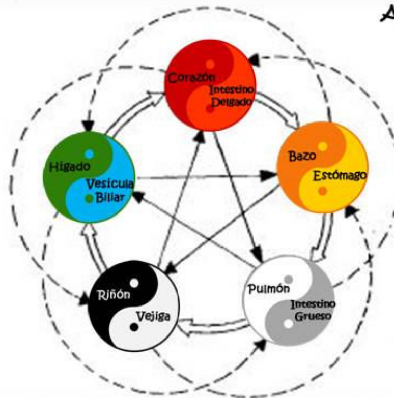
FIG. 2. Relaciones de intergeneración, interdominancia, exceso de dominancia y contra-dominancia entre cinco movimientos: Madera, Fuego, Tierra, Metal y Agua.
