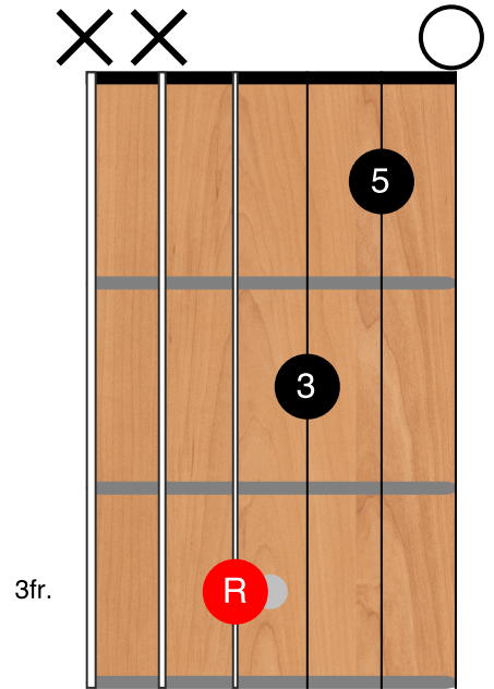
F maj7 Chord
