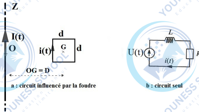
Figure 7 – Influence magnétique éclair-cadre
